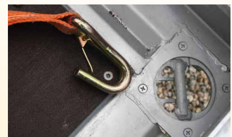
Sonderausstattung: Drehbarer Zurrstab - 1.250 daN (nur in den Ecken möglich)
